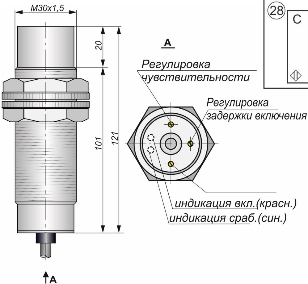
Габаритный чертеж
