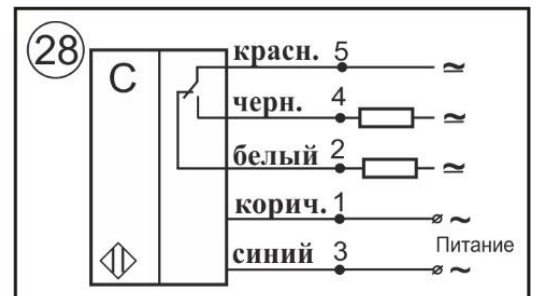
Схема соединения
