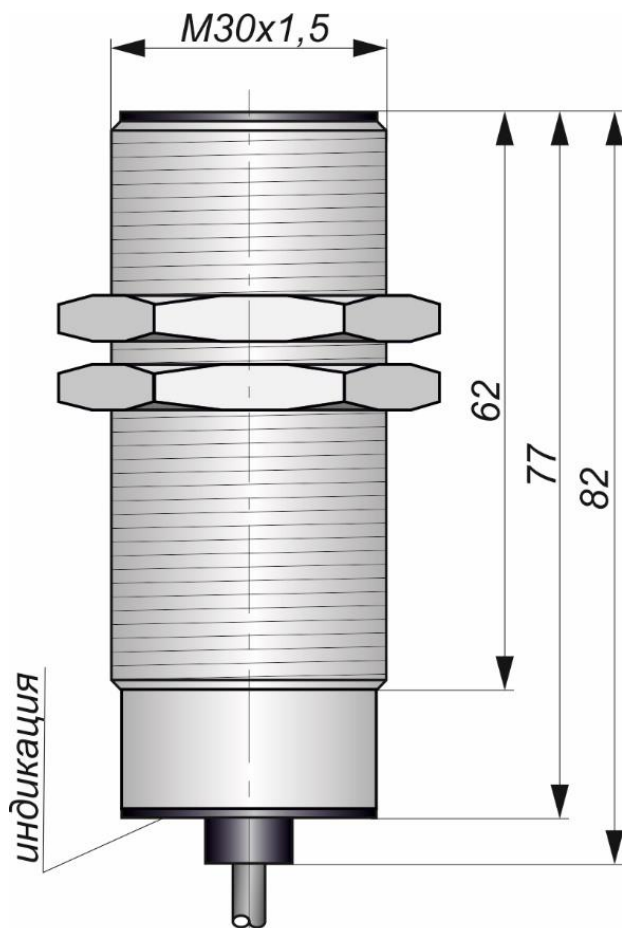
Габаритный чертеж
