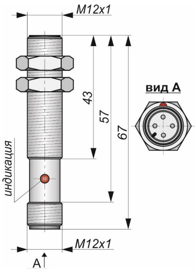
Габаритный чертеж
