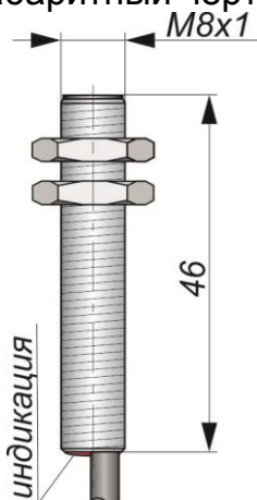
Габаритный чертеж
